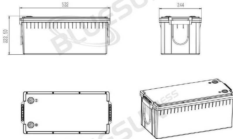
Таблиця 2-1 Розміри пристрою BSM12280
