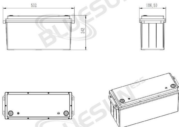
Таблиця 2-1 Розміри пристрою BSM12208
